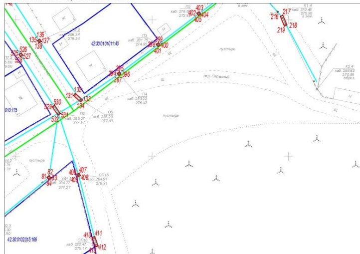
Выносной лист 5-2, масштаб 1:1000
