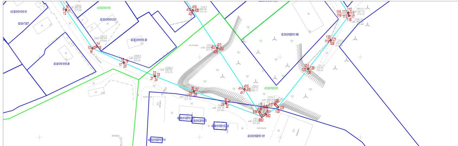
Выносной лист 5-2, масштаб 1:1000
